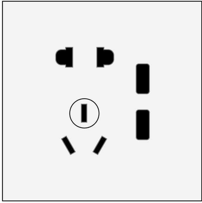
USB五孔插座面板
